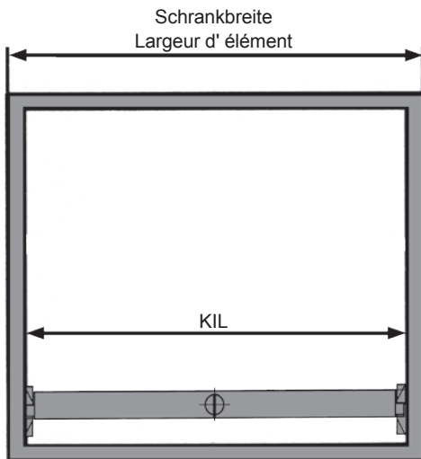
Masszeichnung Dessin de la mesure
