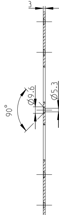
Schließblech 9-29558-00-0-1
