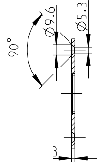
Schließplatte 9-38551-01-0-8
